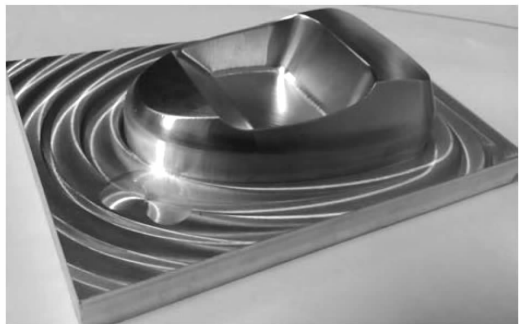
图 6 采用新方法加工后的零件
