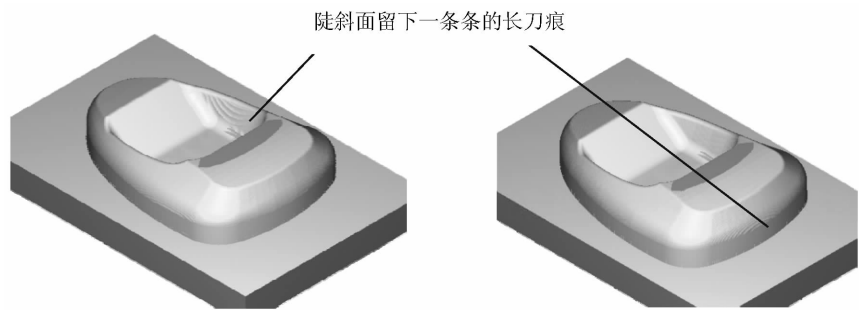
图 4 平行铣削加工 (左图和右图分别走 0° 和 90° 方向)
