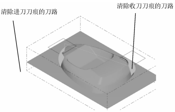
图 5 清除对角进刀和收刀刀痕
