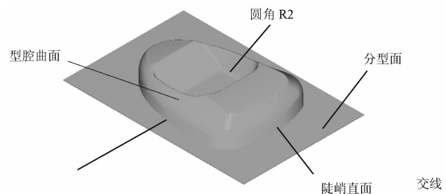
图 1 充电器凸模模型
