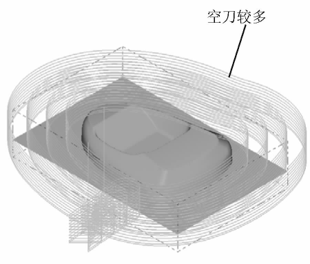
图 2 外形轮廓加工
